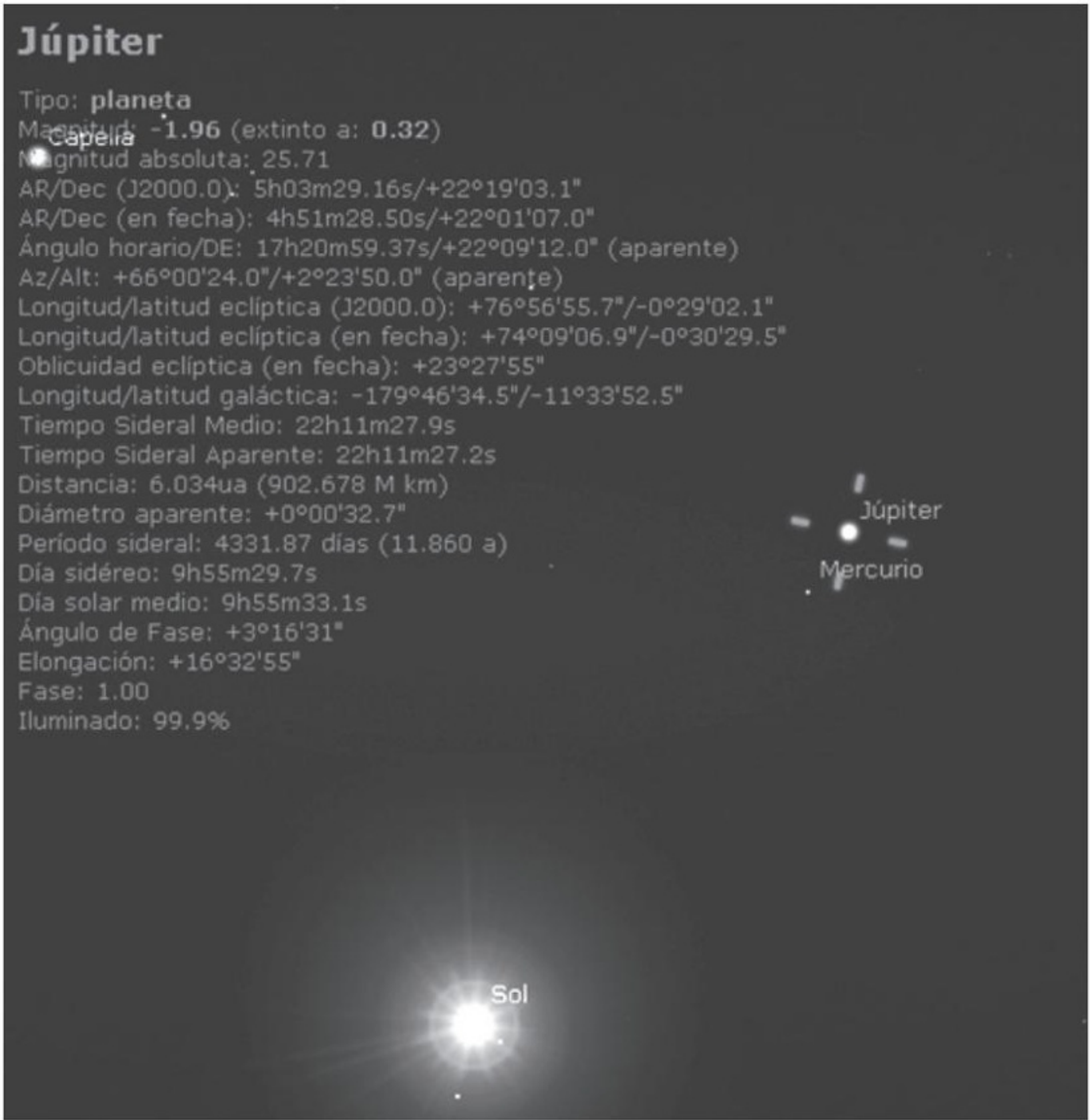
05:10 horas del 22 de junio de 1799, Tenerife. El sol, aún bajo el horizonte, no impide ver una casi conjunción de Júpiter y Mercurio, que fueron las dos “estrellas” que observaron Humboldt y acompañantes en su ascenso al Teide
