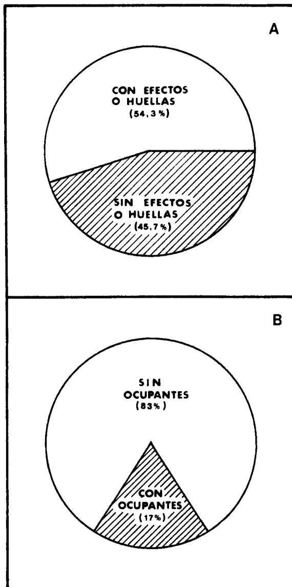
Fig. 4 Proporción de casos con efectos y huellas (A) y con ocupantes (B).
