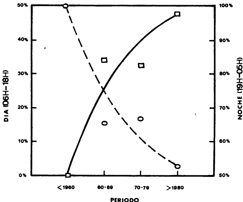
Fig. 3 Observaciones diurnas y nocturnas por décadas.
