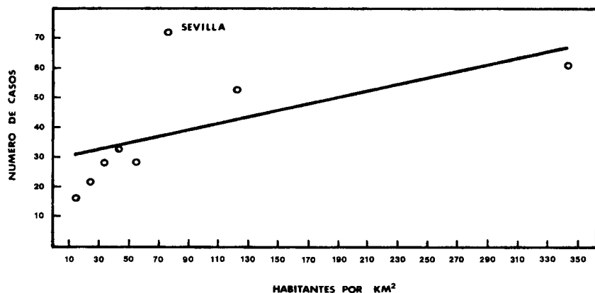
Fig. 6 Recta de regresión lineal.
