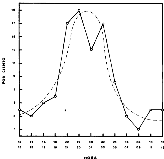
Fig. 5 Porcentaje de casos explicados según la hora del día.
