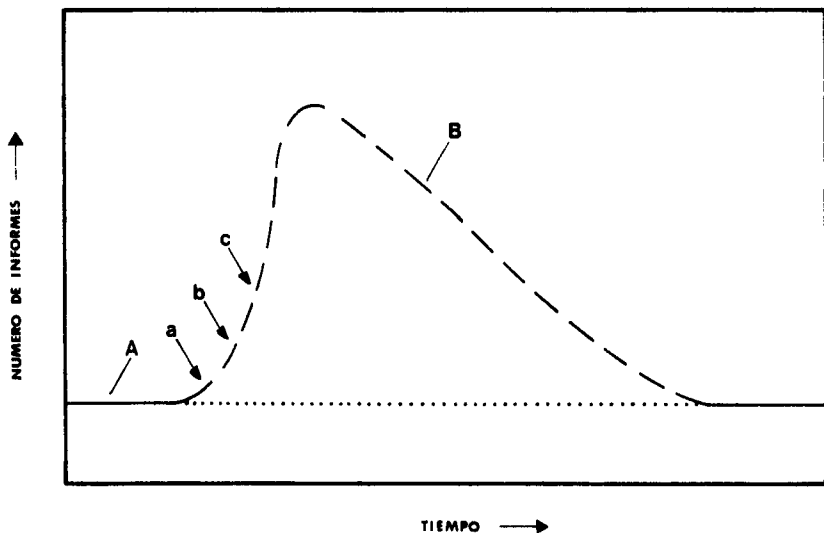
Fig. 7 Modelo teórico del número de informes en el tiempo.
